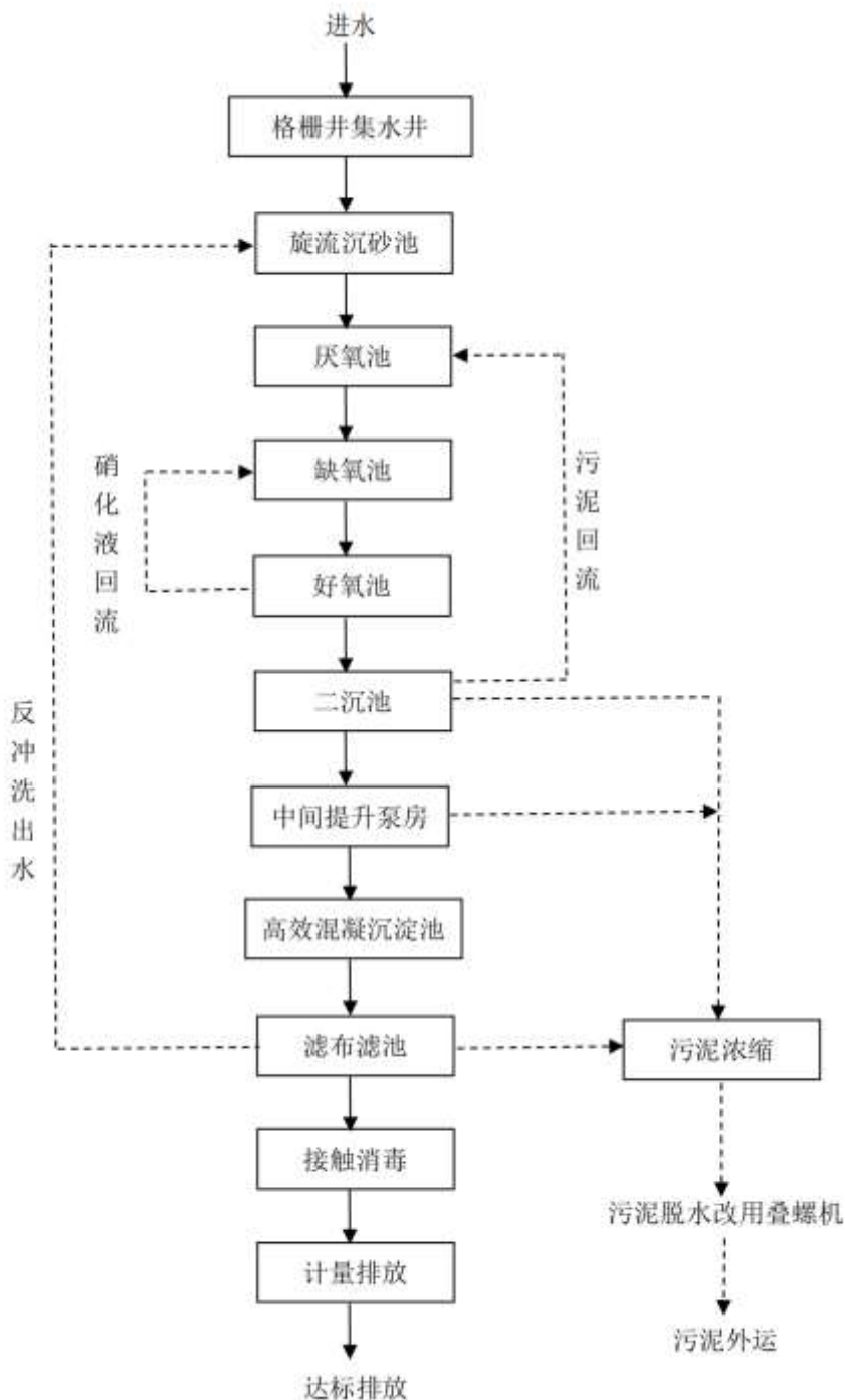
图 2-1 东海县白塔埠镇联村生活污水处理厂污水处理工艺流程
