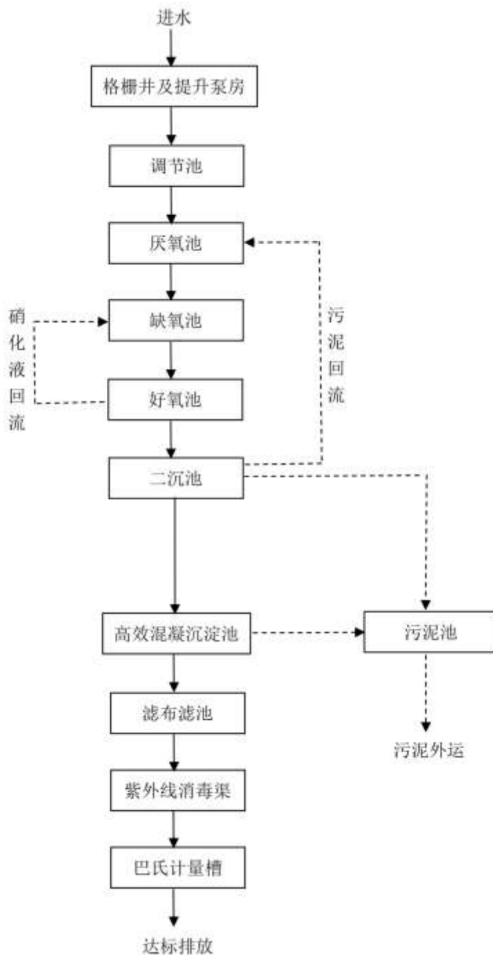
图 2-2 东海县黄川镇王庄村生活污水处理厂污水处理工艺流程
