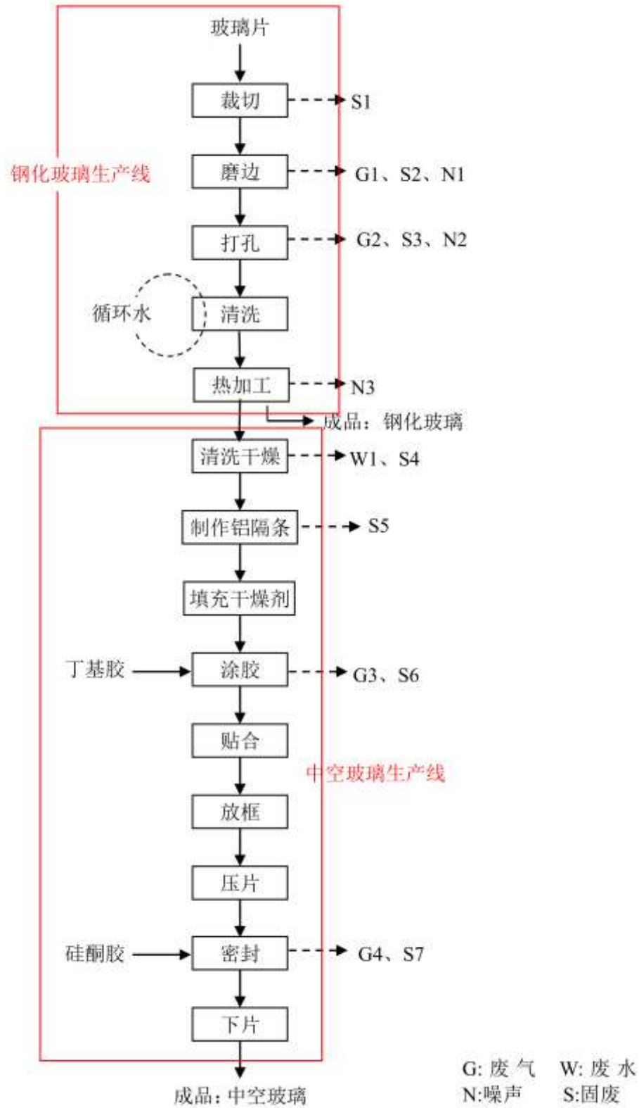
图 2-2 钢化玻璃、中空玻璃生产工艺流程及产污示意图
